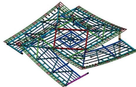
屋面钢结构模型示意图
